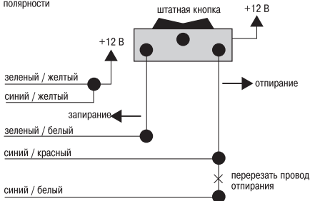
5 - проводная система центрального замка с управлением запираемостью дверей по плюсу и отпиранием дверей импульсом переменной полярности
