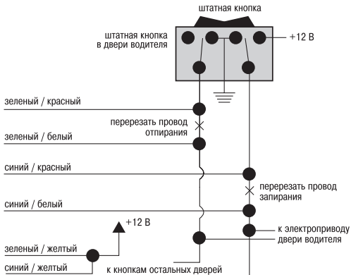
5 - проводная система центрального замка переменной полярности
