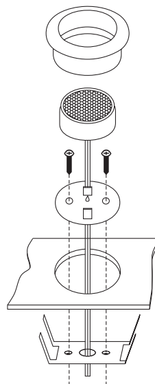
врезка
